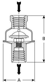
Ableiter Modell WMT-1
