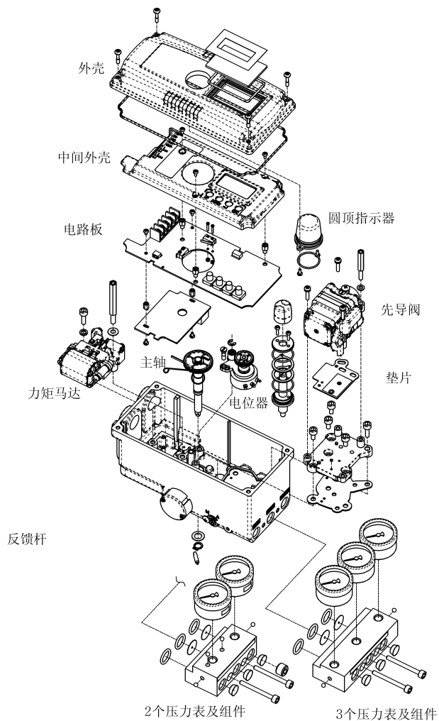
图：YT-3300L结构图
