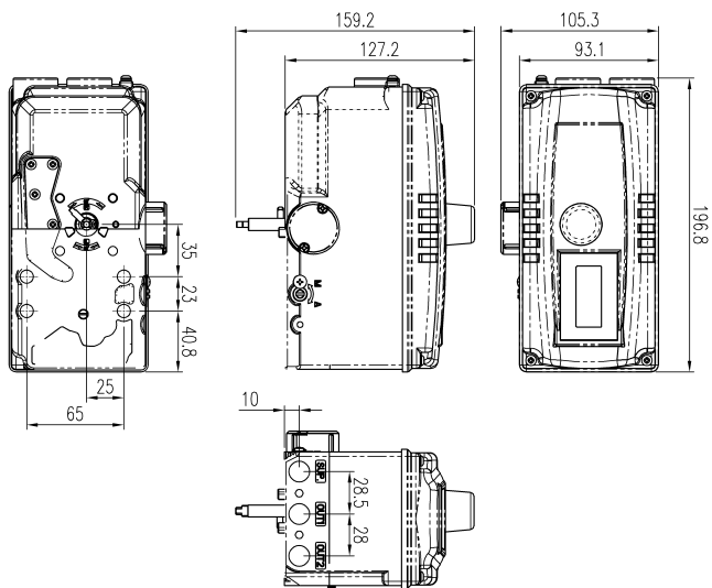
图：YT-3300R 带限位开关型外形图
