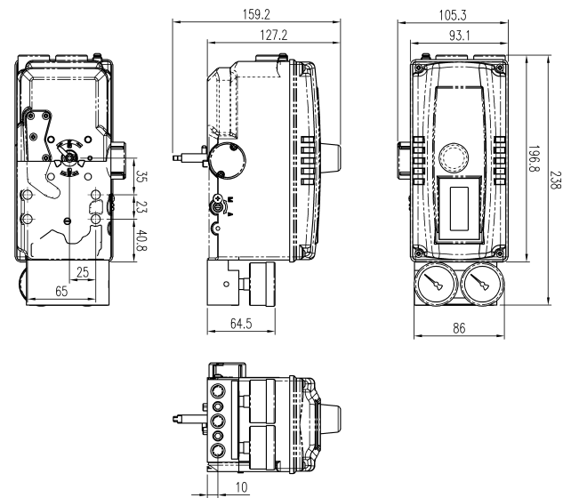
图：YT-3300R 带限位开关及2个压力表外形图
