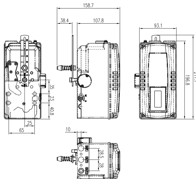
图：YT-3300L外形图
