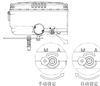
图：自动/手动开关调节
