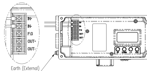
图：YT-3300接线端子
