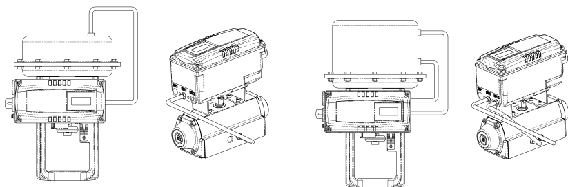
图：执行机构的气管连接例图
