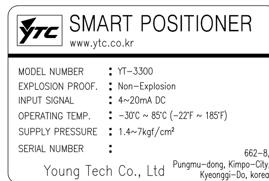
图：产品铭牌图样
