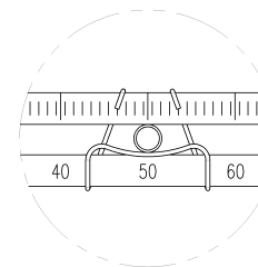
图：连接棒正确连接在反馈杆和固定弹簧上的示意图
