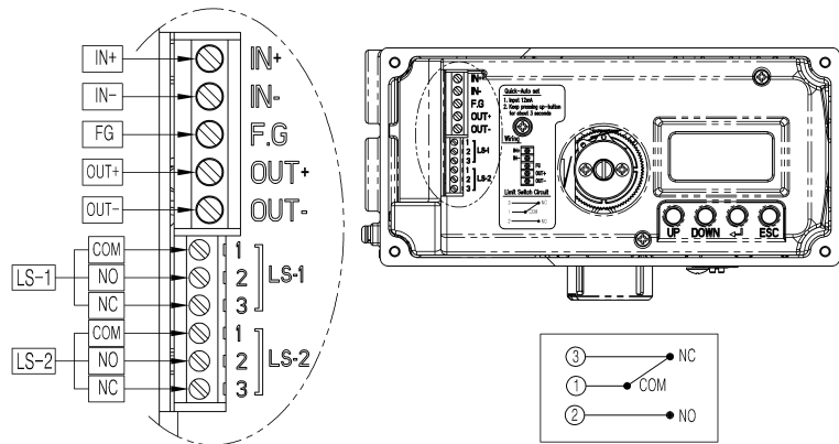
图：机械式开关
