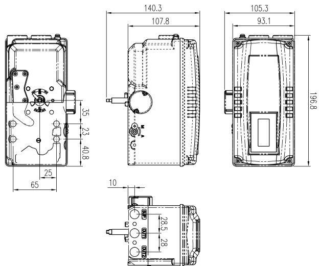
图：YT-3300R 标准型外形图
