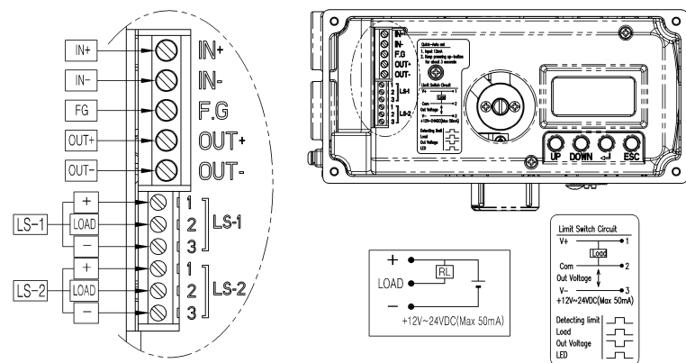
图：感应式开关
