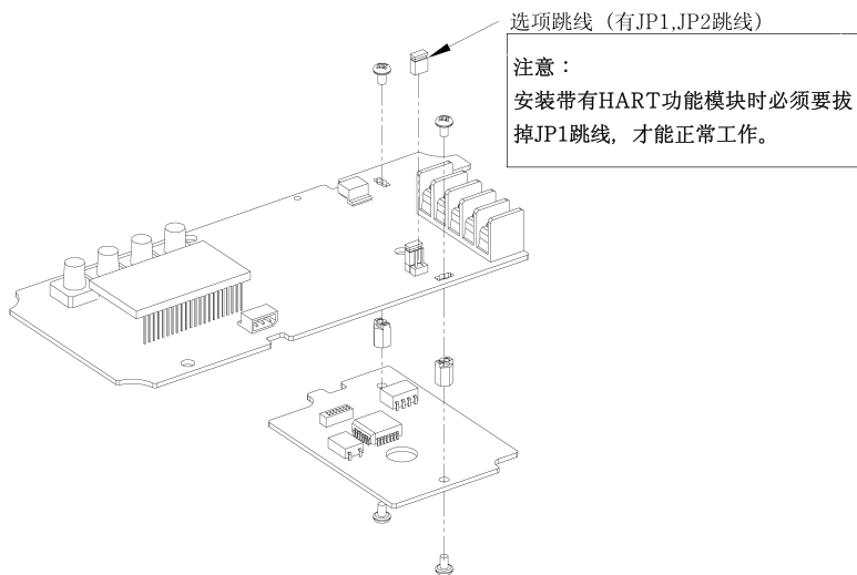
图：选项模块电路板的安装方法
