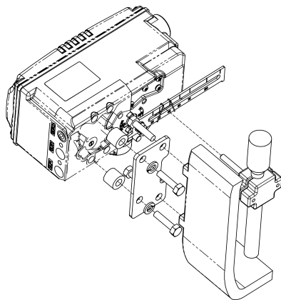
图：YT-3300L 和支架连接图
