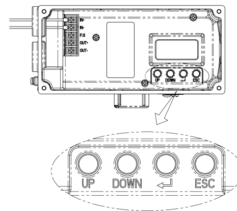
图：打开YT-3300外壳后，从正上方的俯视图
