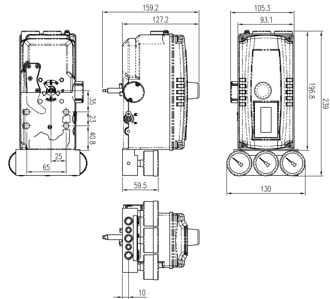
图：YT-3300R 带限位开关及3个压力表外形图
