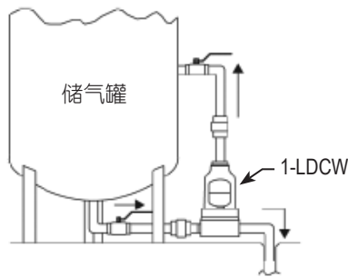
图 1. 排液阀需安装在储气罐下方，排气平衡口需连接至储气罐内液位以上的位置。
