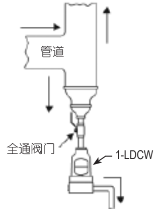
图 6. 排液阀用于排出压缩空气分配管中的液体。
