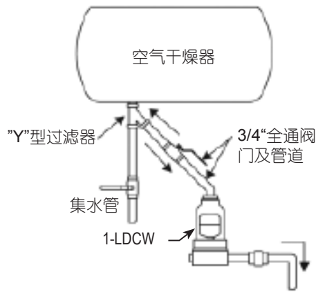
图 7. 排液阀用于排出少量液体，使用上部平衡口作为进水口，需要采用3/4"进水管，选用全通阀门（例如：球阀或闸阀等），进水管尽可能缩短并在安装排液阀前将所有配件吹扫干净。
