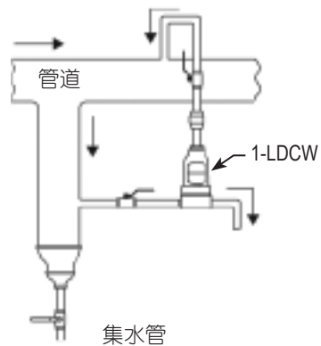
图 4. 排液阀用于排出水平压缩气输气管中的液体。
