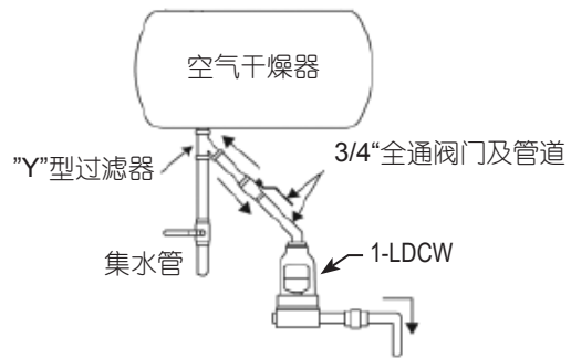
图 2. 排液阀安装在干燥器下方，使用顶部平衡口作为进水口，需要采用3/4英寸进水管，选用全通阀门（例如：球阀或闸阀等），进水管尽可能缩短并在安装排液阀前将所有配件吹扫干净。
