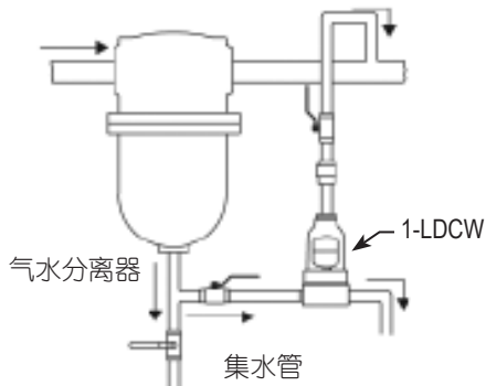
图 3. 排液阀用于排出气水分离器中的液体。
