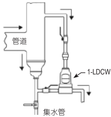
图 5. 排液阀用于排出压缩空气分配管中的液体。
