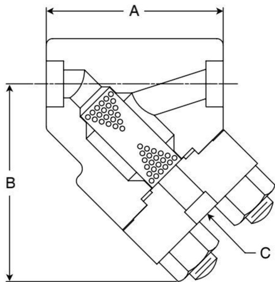
D1SW DN15-50
